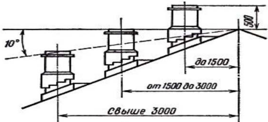
Рис.19 Расположение дымовых (вентиляционных) труб относительно конька крыши
