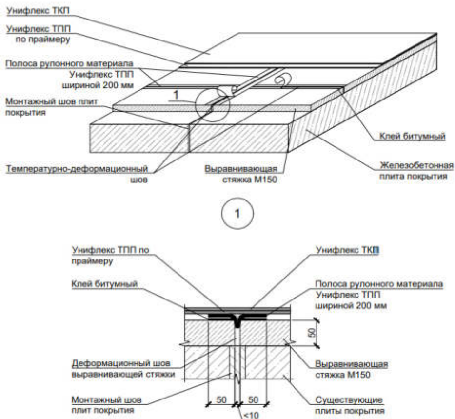
Рис. 22 Схема температурно-усадочного шва
