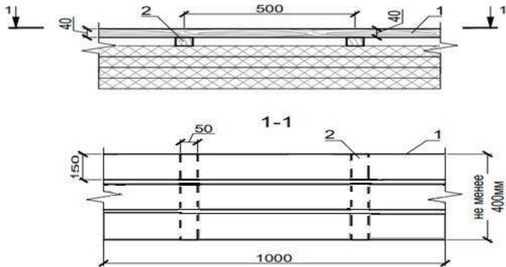
Рис. 25 Вариант устройства ходовых трапов в чердачном помещении
