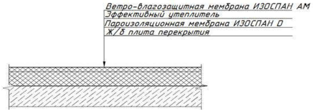
Рис. 27 Утепление чердачного перекрытия железобетонного (плоские плиты)
