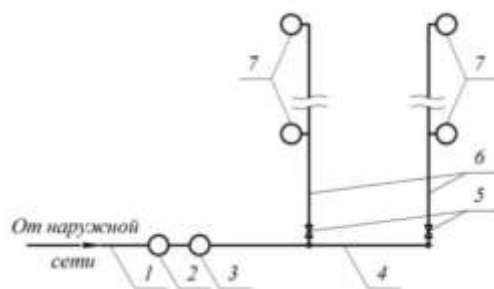
Рис. 7 Схема внутреннего водопровода МКД
