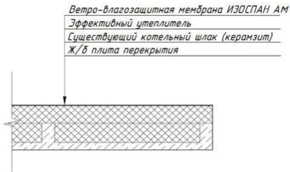
Рис. 26 Утепление чердачного перекрытия железобетонного (ребристые плиты)
