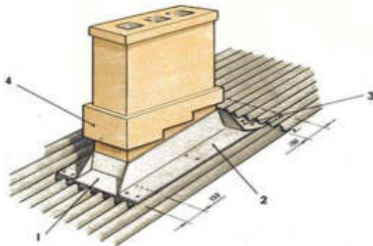
Рис. 20 Примыкание к вентиляционным трубам
