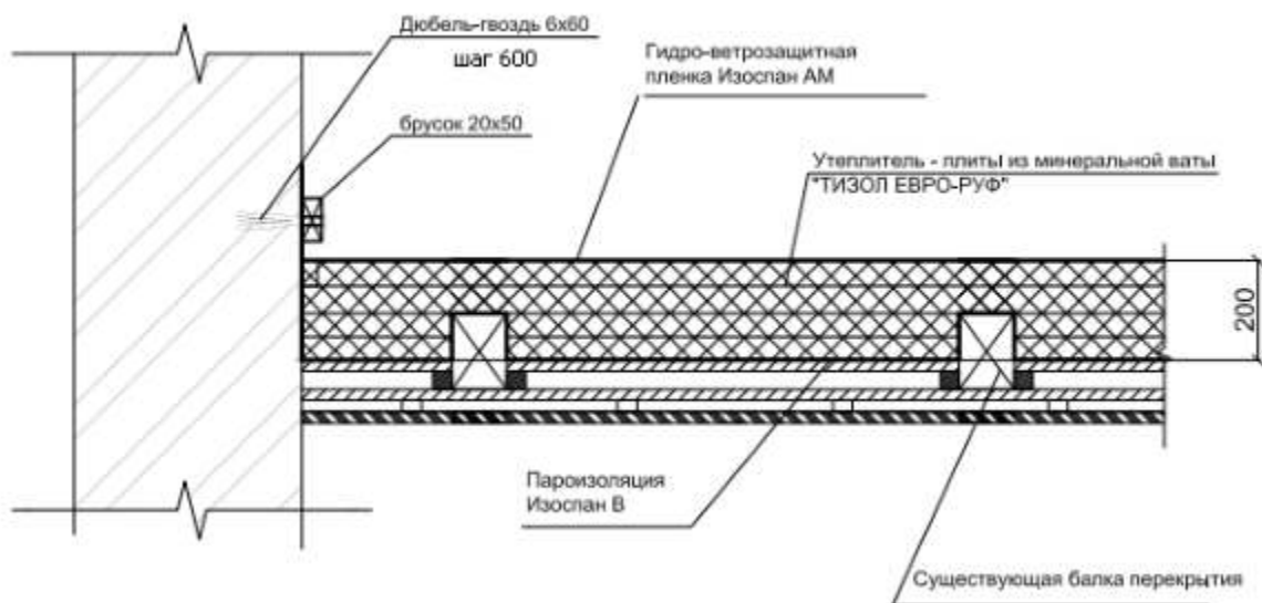
Рис. 23 Крепление пароизоляции, гидро – ветрозащитной мембраны
