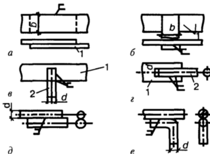
Рис. 5 Соединение заземляющих проводников с горизонтальными заземлителями: а) - продольное соединение проводников из полосовой стали; б) - ответвление проводника из полосовой стали; в) - ответвление проводника из круглой стали; г) - продольное соединение проводников из полосовой и круглой стали; д) - продольное соединение проводников из круглой стали; е) - ответвление проводника из круглой стали: 1 - стальная полоса, 2 - сталь круглая
