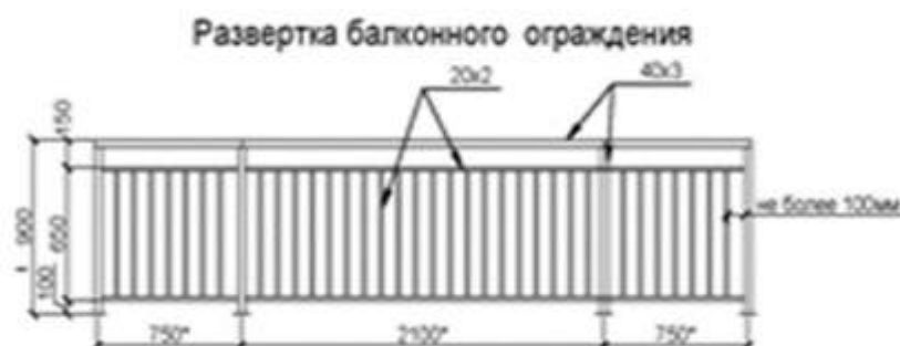
Рис. 28 Развертка балконного ограждения
