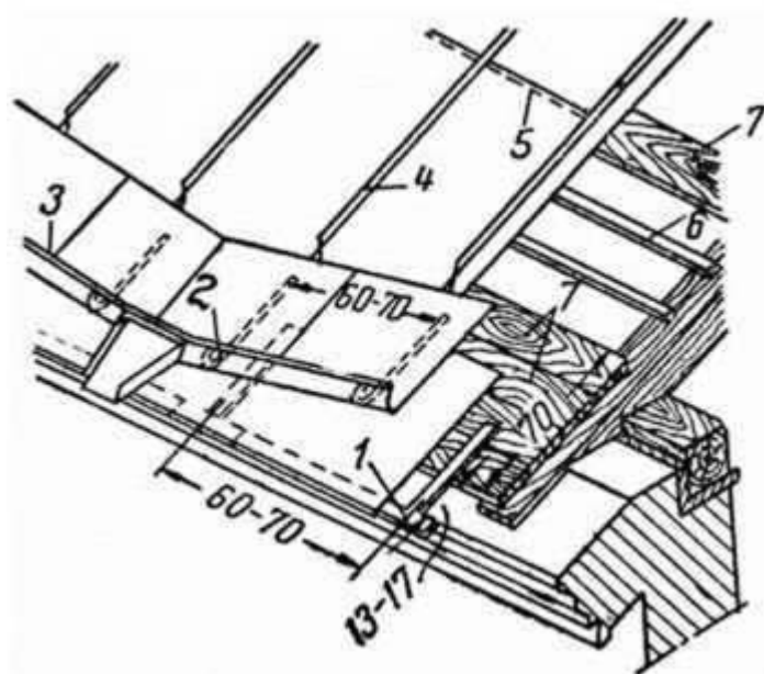
Рис.13 Элементы кровли из листовой стали
