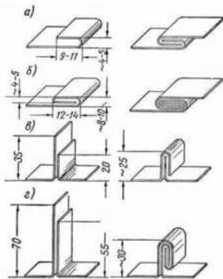
Рис. 14 Способы соединения картин кровельной стали (размеры в мм)
